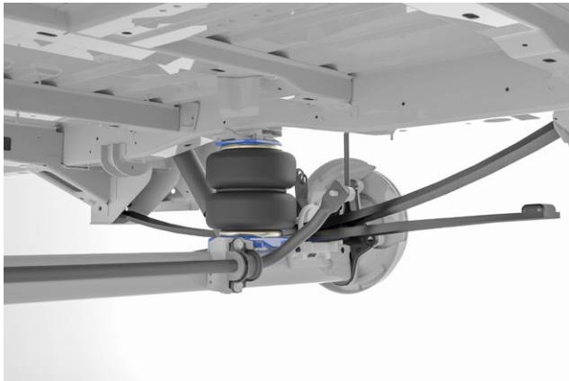
SATZFOTO: BLATTFEDERUNG
